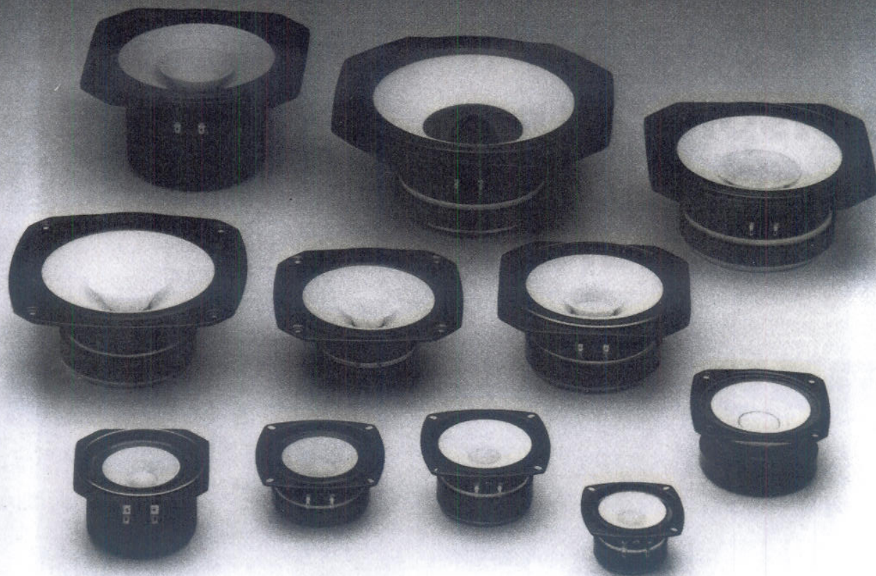
■ Obere Reihe: FE206Σ, FP253, FP203 ■ Mittlere Reihe: FE204, FE164, FP163 ■ Untere Reihe: FE106Σ, FE103, FE103Σ, FE83, FE127
